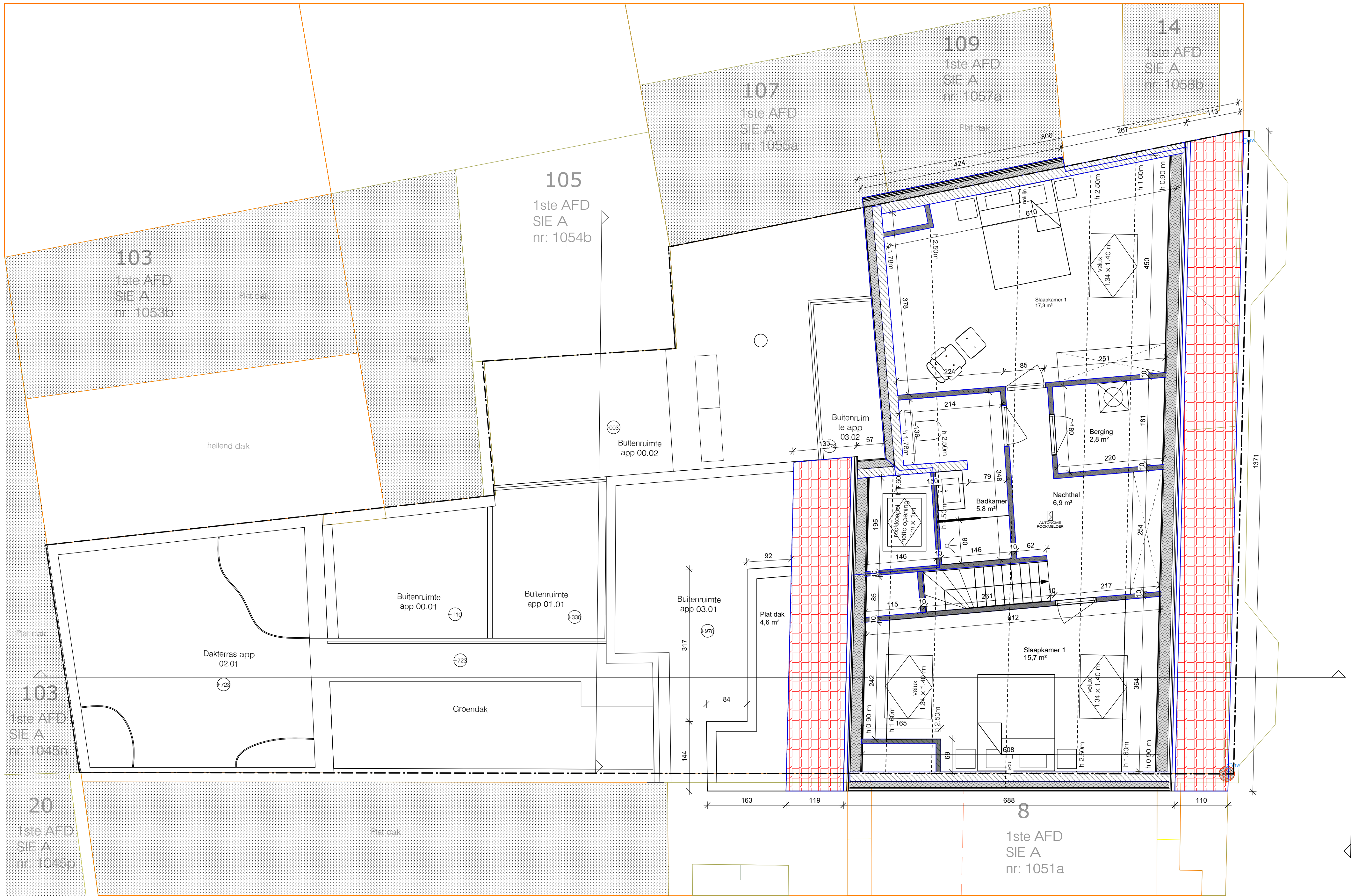
Grondplan dakverdieping
